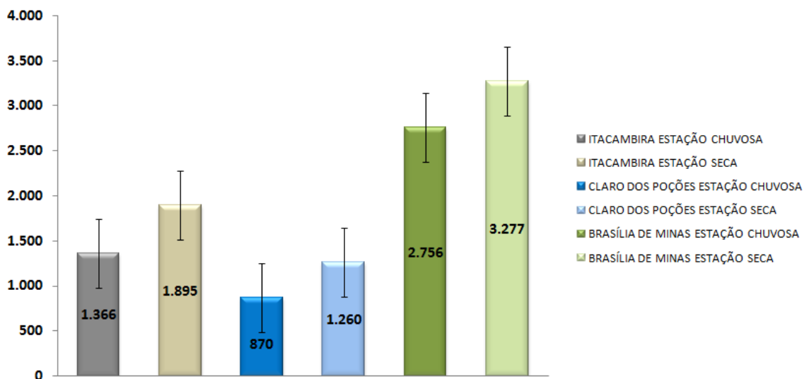
Fig.1 Abundância média de esporos em função das cidades amostradas - Itacambira, Claro dos Poções e Brasília de Minas mostrando as estações chuvosa com 1.366, 870 e 2.756 esporos e seca com 1.895, 1.260 e 3.277 esporos respectivamente.
